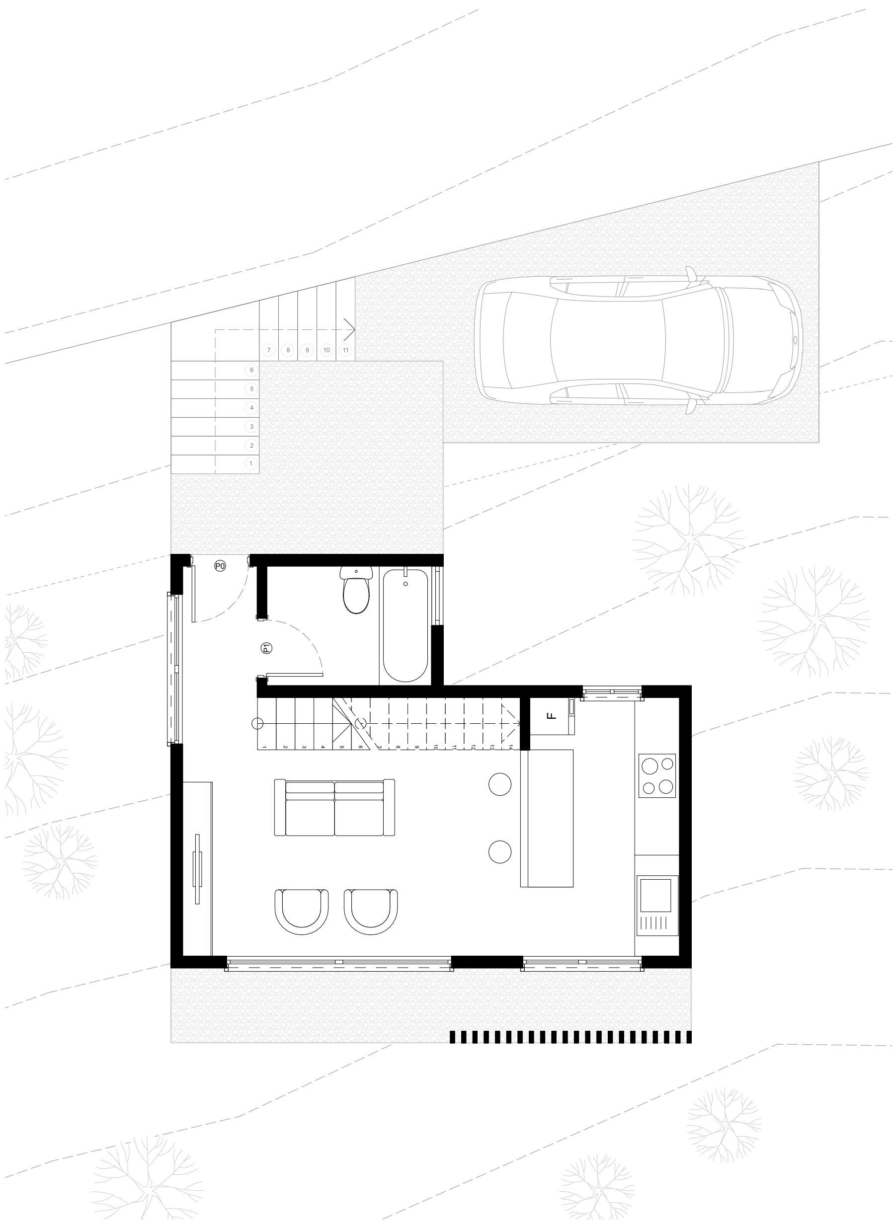
PLANTA NIVEL 1 : 35,75 M2
