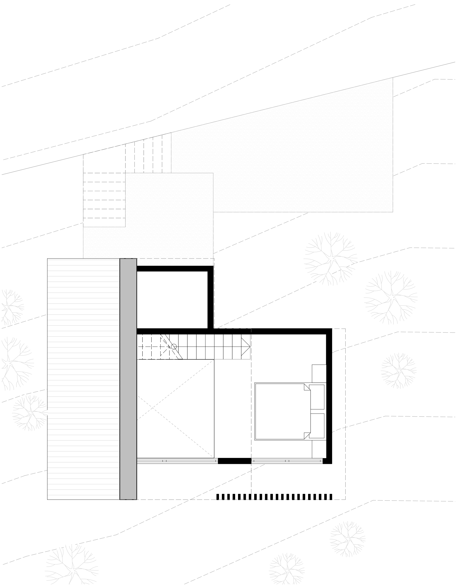
PLANTA NIVEL 2 : 14,02 M2
