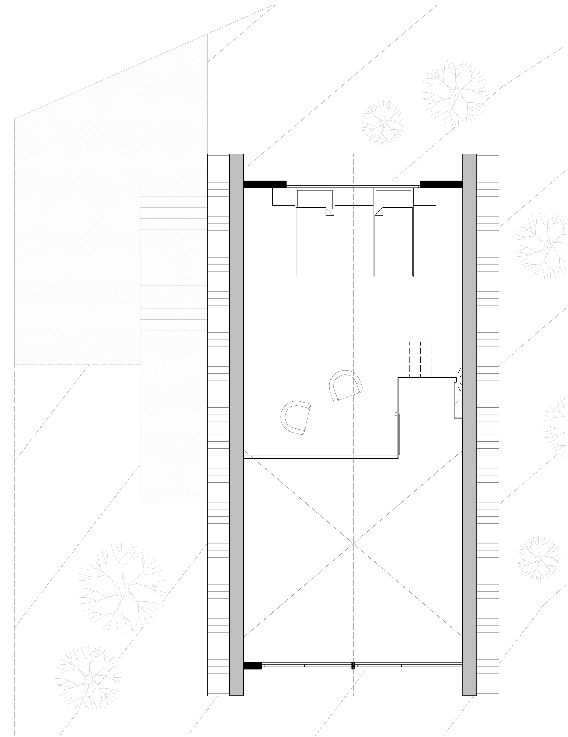
PLANTA NIVEL 2 : 22,22 M2
