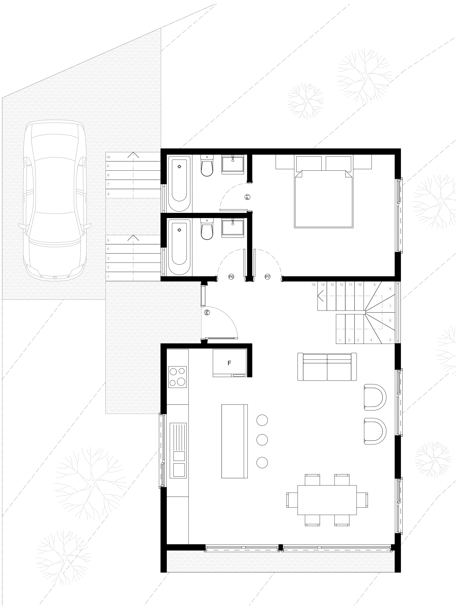
PLANTA NIVEL 1 : 73,75 M2
